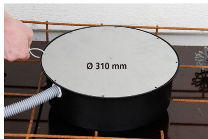
Werkzeuglose und absolut betondichte Einführung für Kabel oder die Rohrgrößen M20 und M25.
