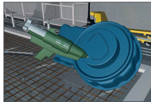
XL Flexgroszdose mit Heißkleber auf den Schaltisch kleben.
