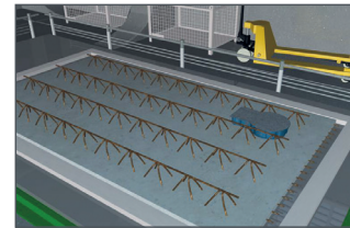
Betonfertigteil wird gegossen.
